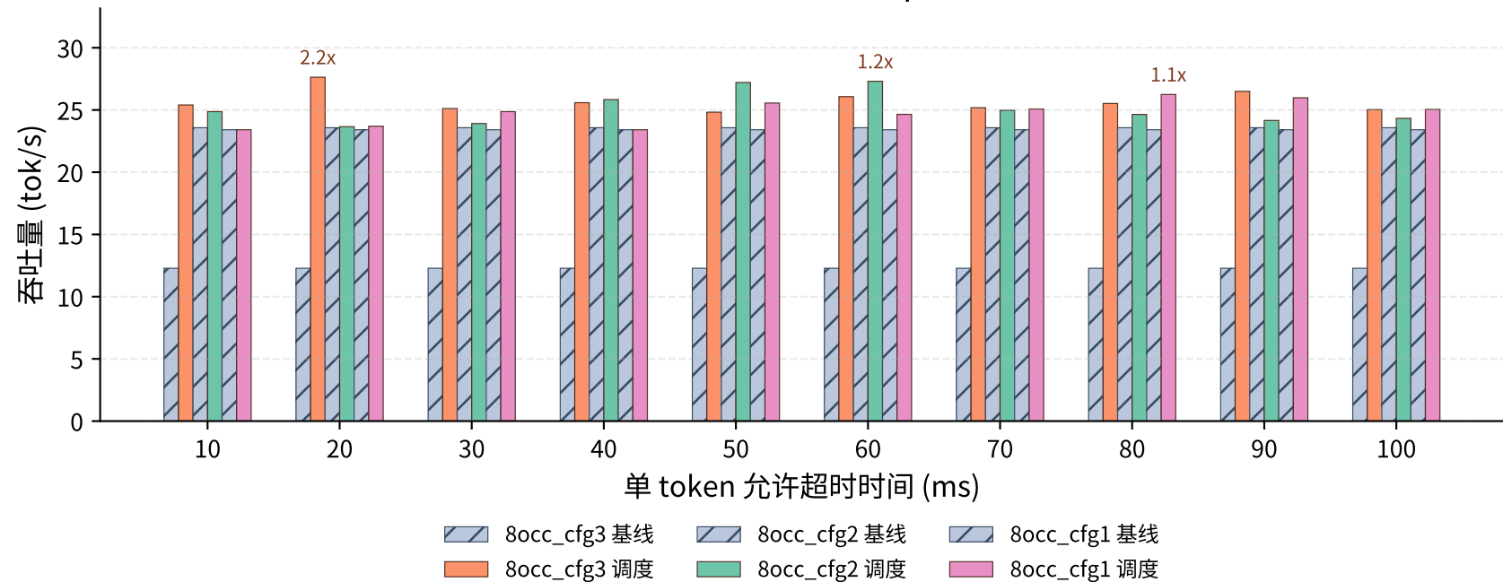
8 核可用，8 核有占用：Top-3 提速配置
