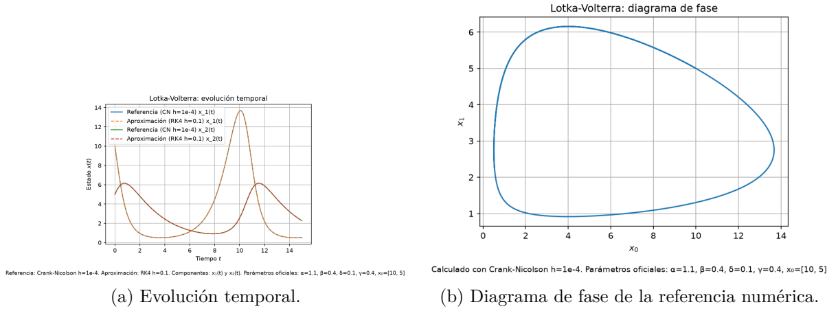
Figura 2: Lotka–Volterra con \alpha = 1.1 , \beta = 0.4 , \delta = 0.1 , \gamma = 0.4 y (x(0), y(0)) = (10, 5) . En (a), RK4 con h = 0.1 se compara con la referencia Crank–Nicolson con h = 10^{-4} ; en (b) se muestra la órbita calculada con esa referencia.
