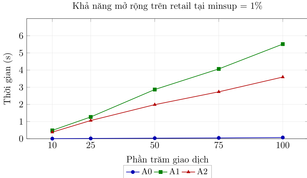
Hình 4.7: Thời gian chạy theo kích thước dữ liệu trên retail (minsup = 1%).
