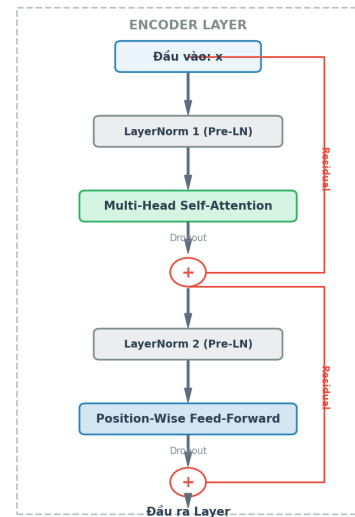
Hình 5: Thiết kế Pre-LN trong một tầng Encoder Layer.
