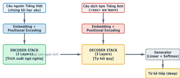
Hình 1: Dòng chảy dữ liệu tổng quát giữa Encoder Stack và Decoder Stack.
