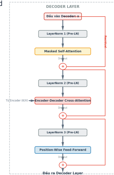
Hình 6: Thiết kế Pre-LN trong một tầng Decoder Layer.
