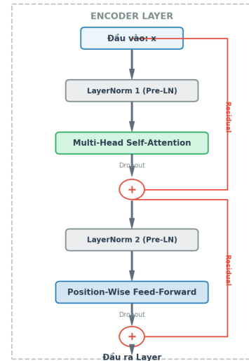
Hình 5: Thiết kế Pre-LN trong một tầng Encoder Layer.
