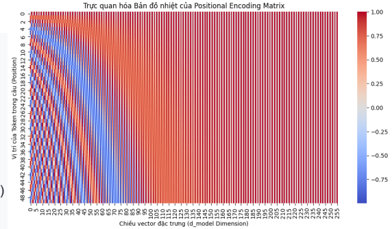
Hình 3: Bản đồ nhiệt trực quan hóa ma trận PE với tần số thay đổi dần theo số chiều.
