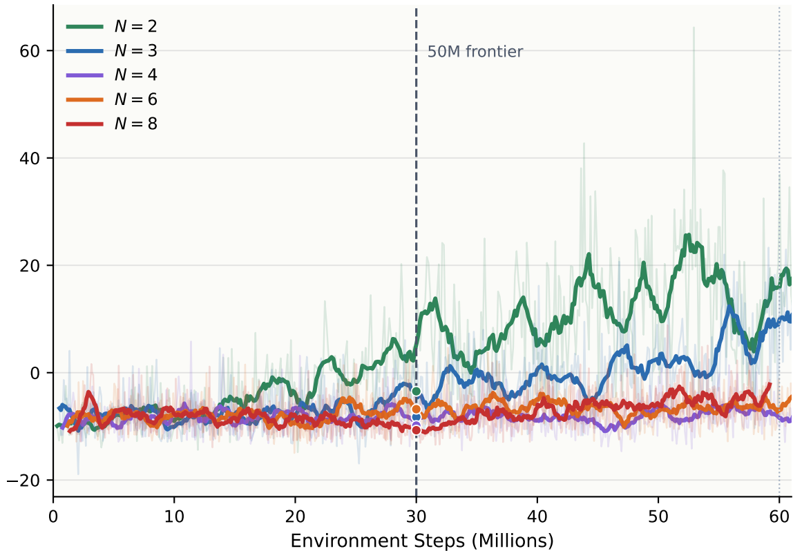
Average shaped episodic return
