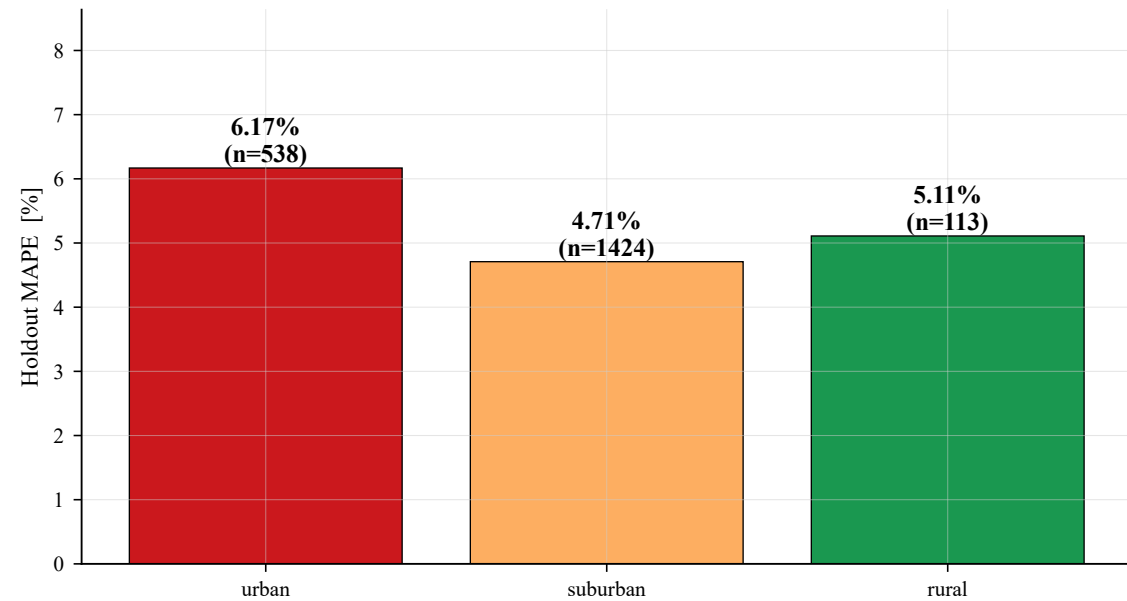
(a) Surrogate-Quality je Raumtyp_3
