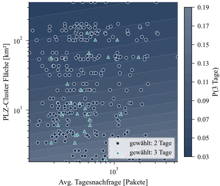
(a) Entscheidungs-fläche P(3 Tage)
