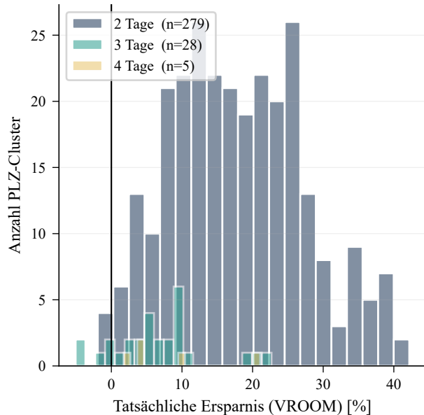
(b) Ersparnis-Verteilung je Schedule-Größe
