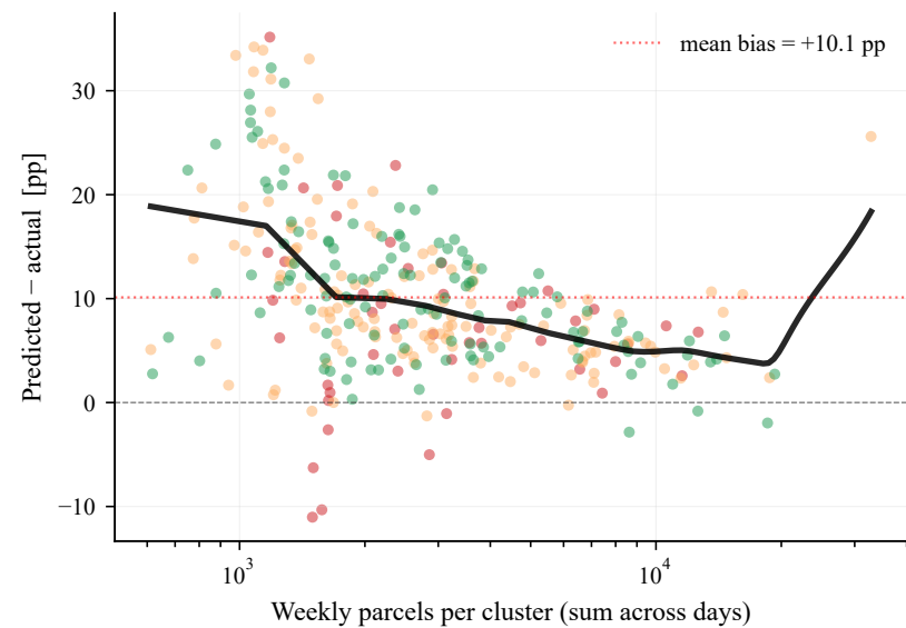
Fig S6 — Surrogate-Bias als Funktion der Features (pp = percentage points)
