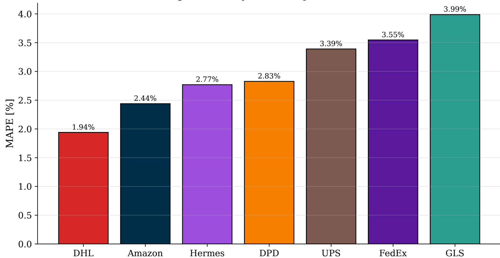
Daganzo-LGB-Hybrid MAPE per LSP (OOF)
