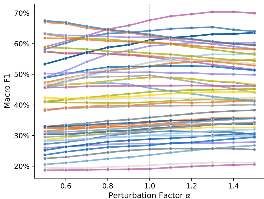
Macro F1
