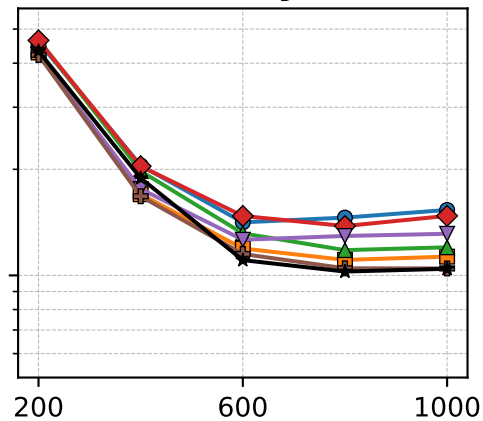
(d) Heavy-hex
