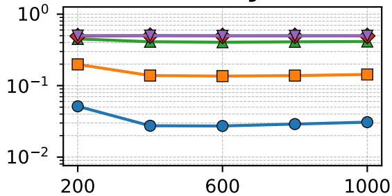
(d) Heavy-hex
