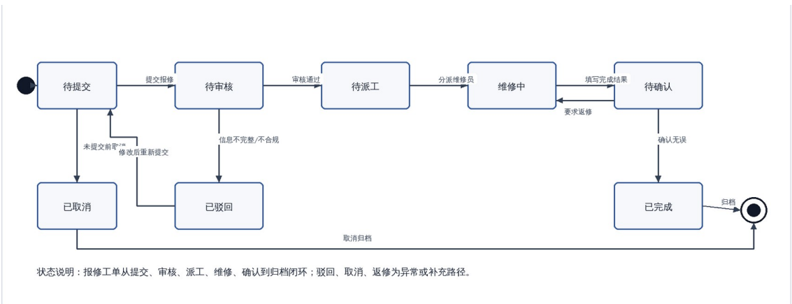
图 4 核心业务状态图
