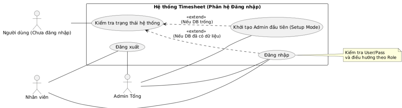
Figure 1: Sơ đồ Use Case phân hệ Đăng nhập
