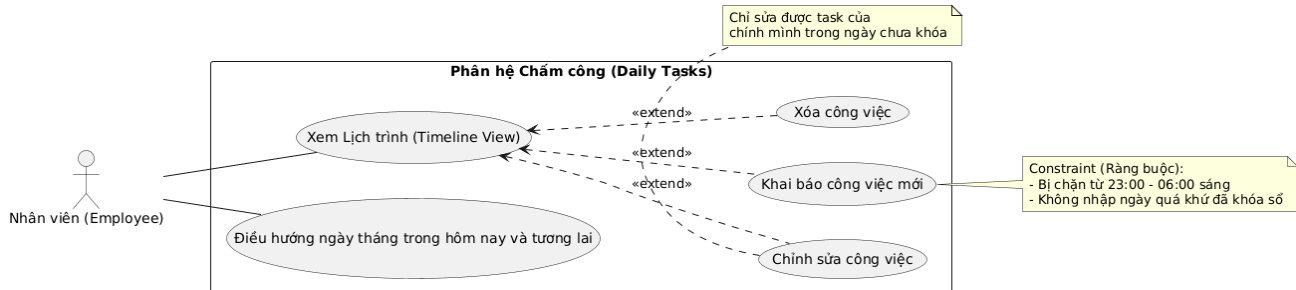
Figure 2: Sơ đồ Use Case phân hệ Chăm công
