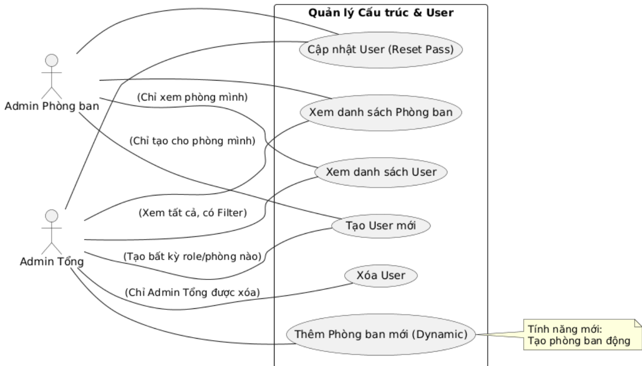
Figure 4: Sơ đồ Use Case quản lý Cấu trúc &amp; User
