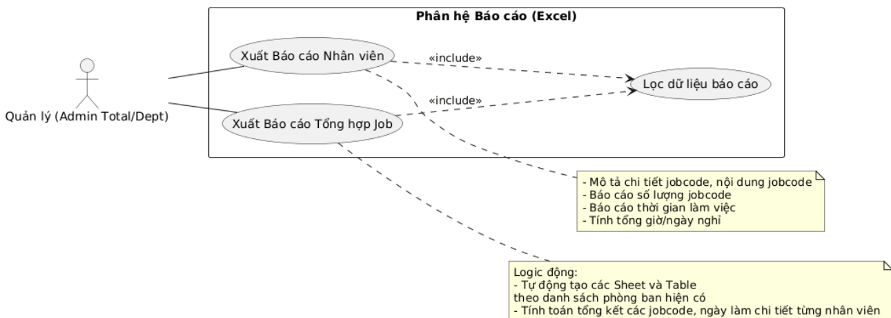
Figure 5: Sơ đồ Use Case phân hệ Báo cáo
