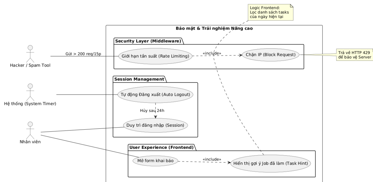
Figure 6: Sơ đồ các tính năng Bảo mật và Tiện ích bổ sung
