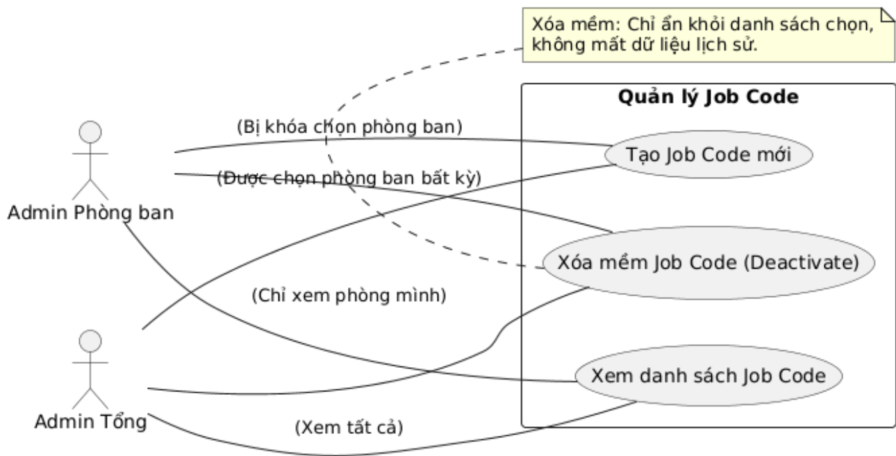
Figure 3: Sơ đồ Use Case quản lý Job Code
