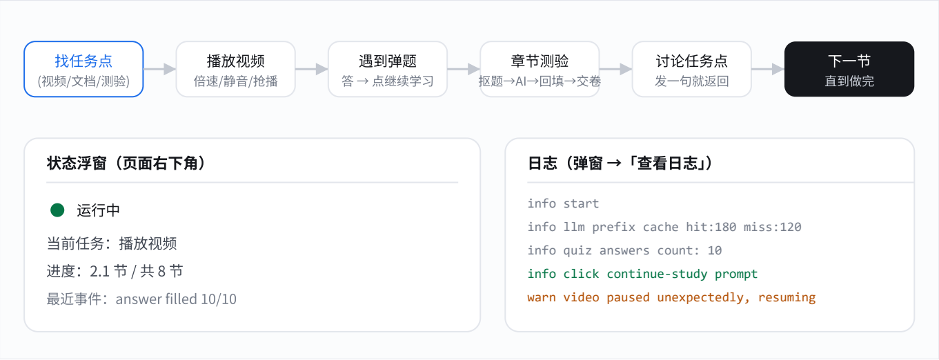
图 3 一次刷课的流程，以及两个观察窗口：状态浮窗看"在干什么"，日志看"为什么"
