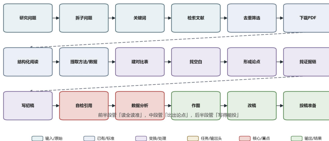
图 19 科研 Agent 完整链路
