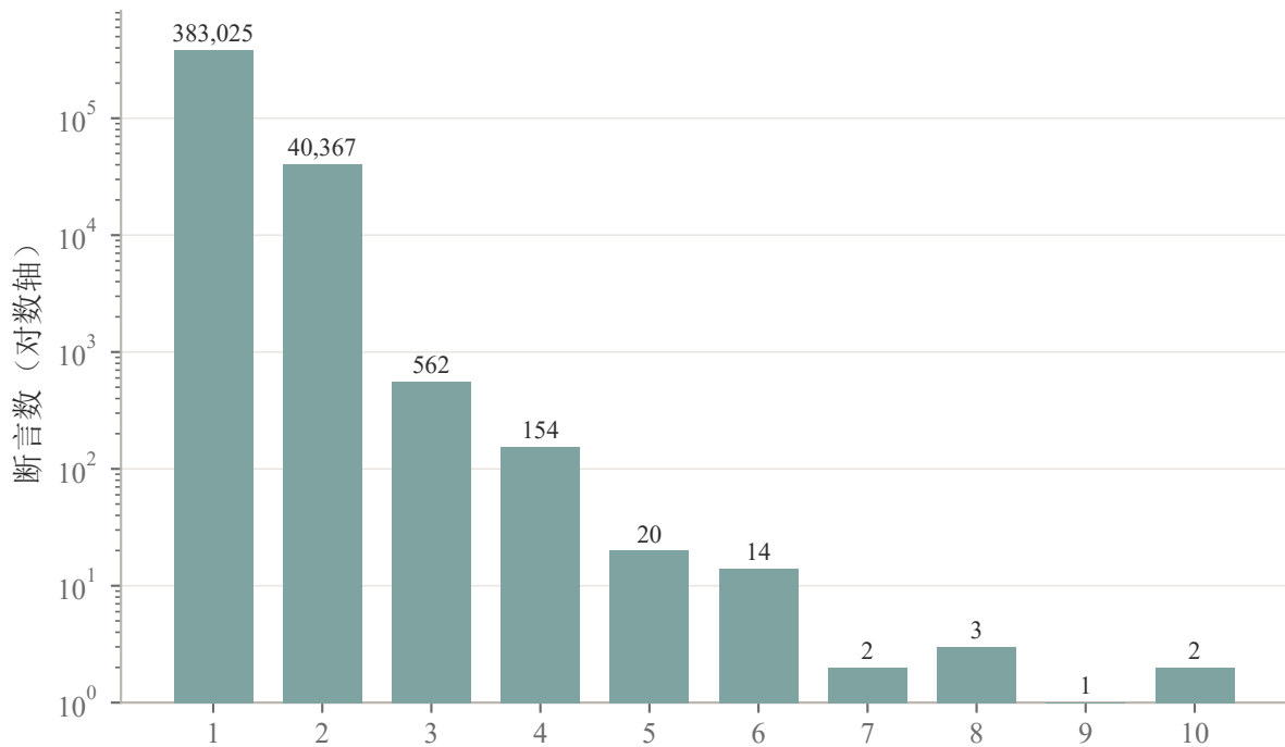
A07 来源成员数分布
