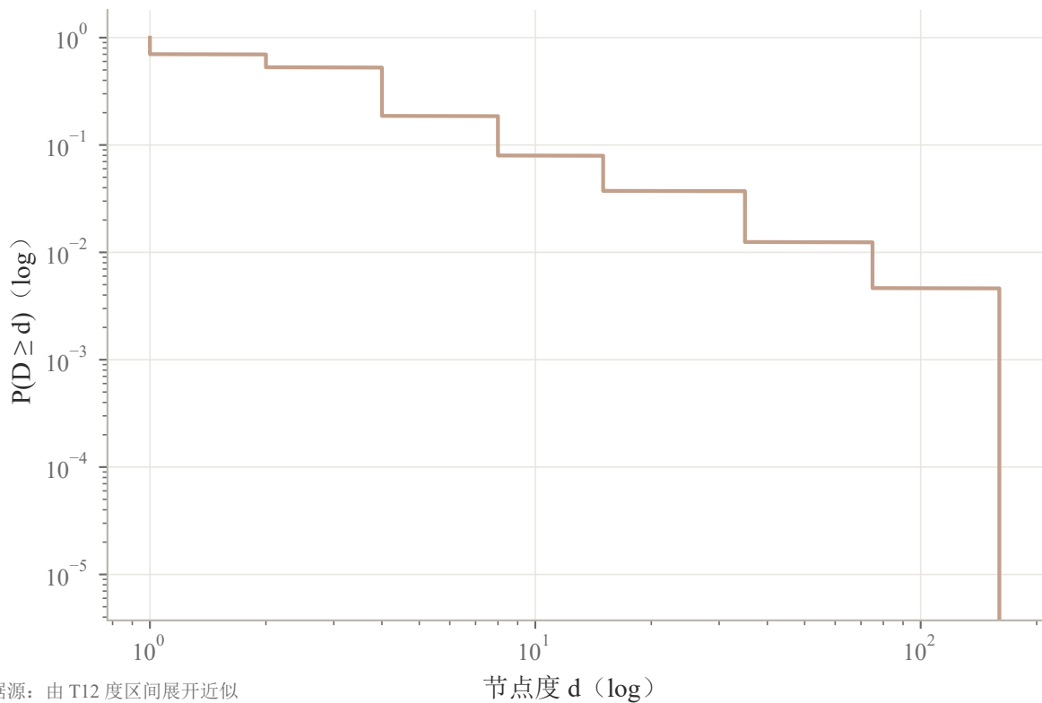
度分布互补累积函数 (CCDF)
