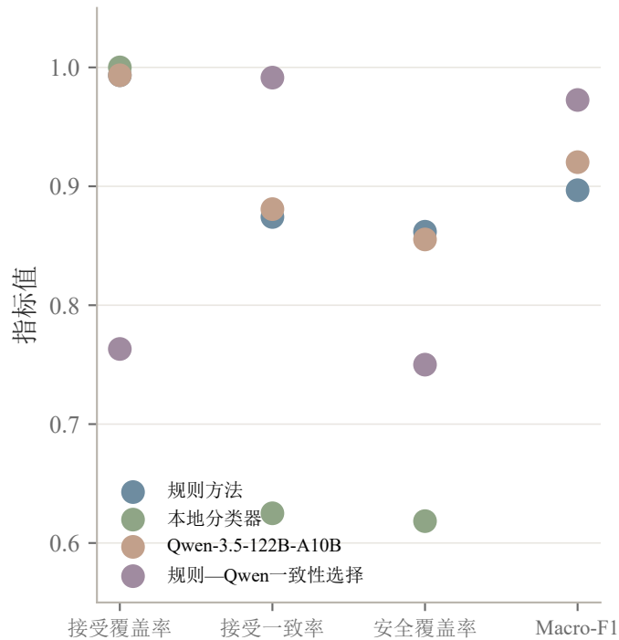
(c) 四种语义判定方法对比 (n=152 核心评价)
