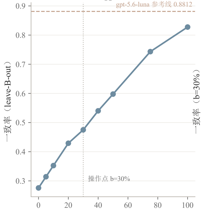
(a) 预算-质量曲线 (gpt-oss-20b 同模型)
