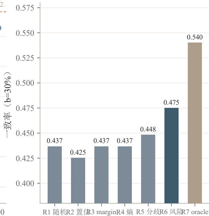
(b) 七种路由策略对比 (R6 判语: 略优)
