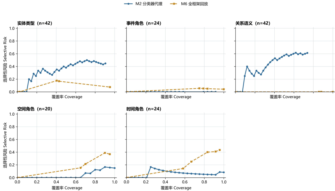
约束选择推断的风险—覆盖曲线（冻结集成参考标注测试集）
