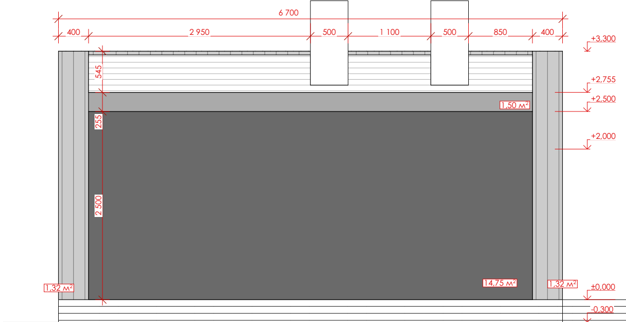
Фасад 4
