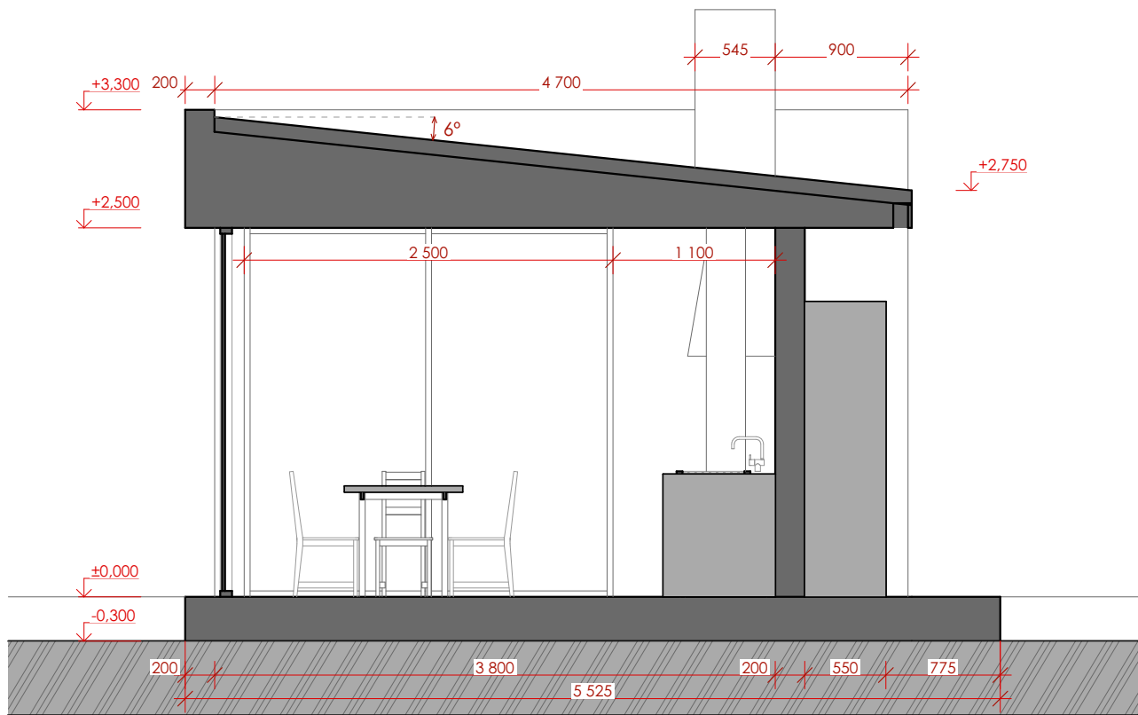
Разрез 3-3
