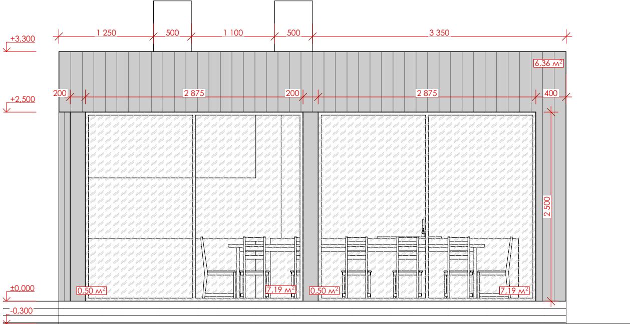
Фасад 2
