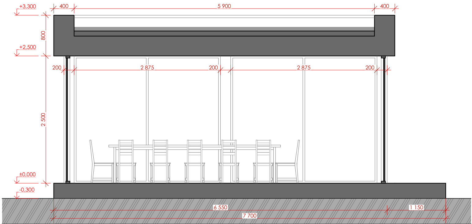
Разрез 4-4
