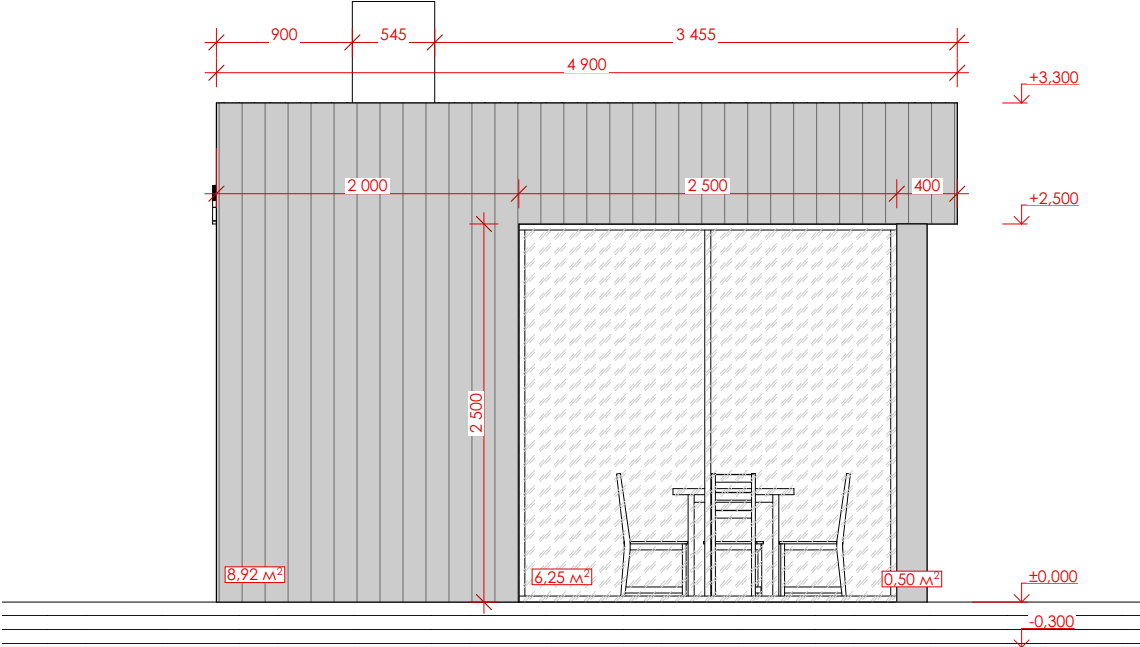
Фасад 3
