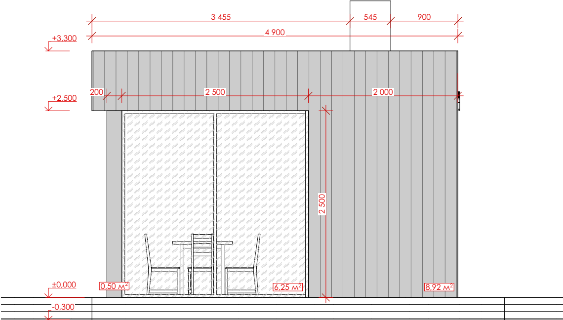
Фасад 1
