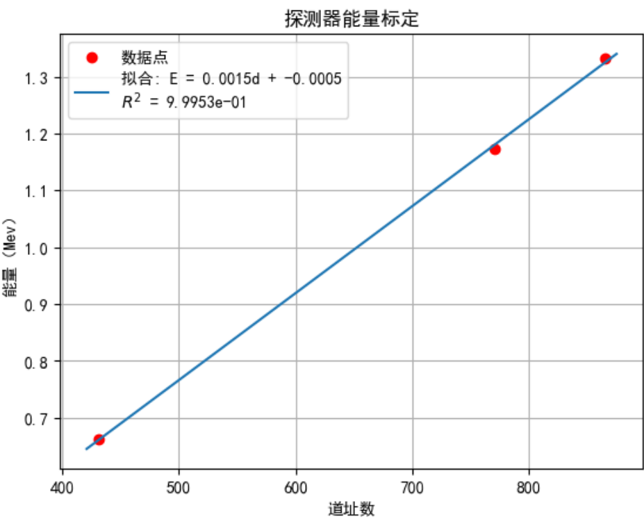
图 4: 对探测器进行能量标定
