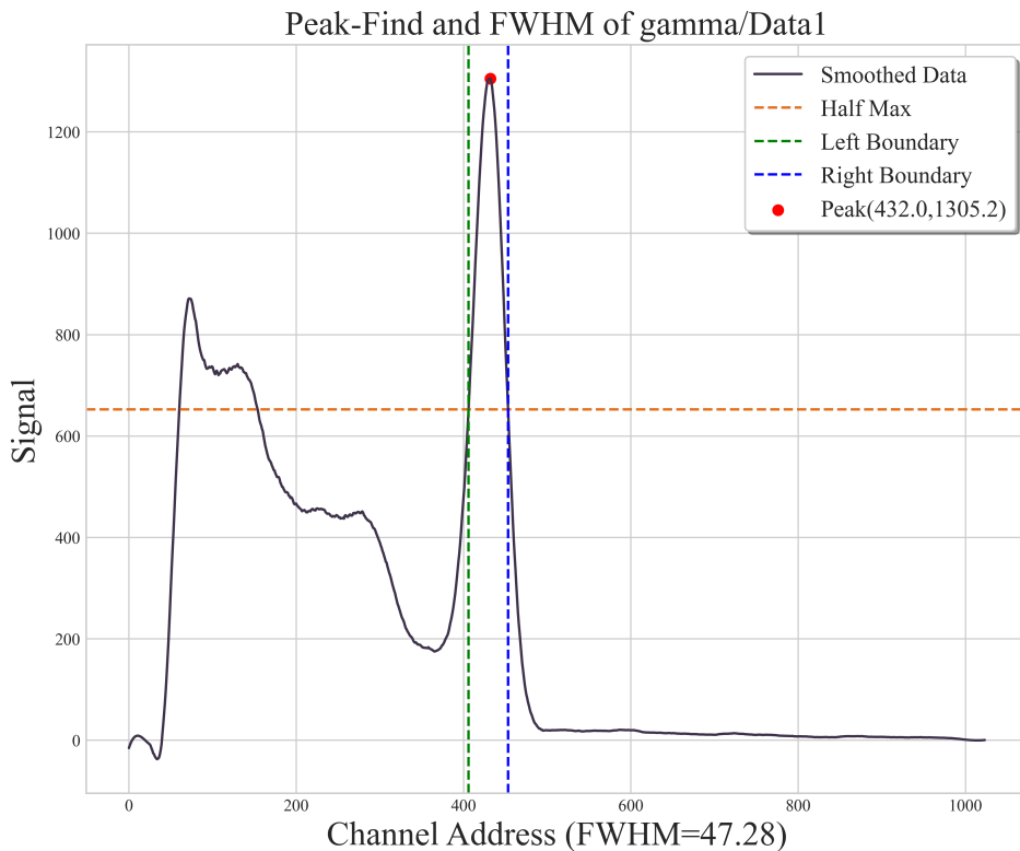
图 5: ^{137}\text{Cs} 主峰与全高半宽
