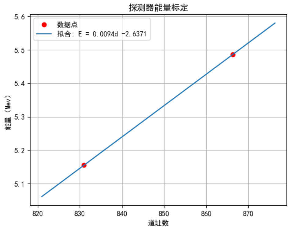
图 10: 对探测器进行能量标定
