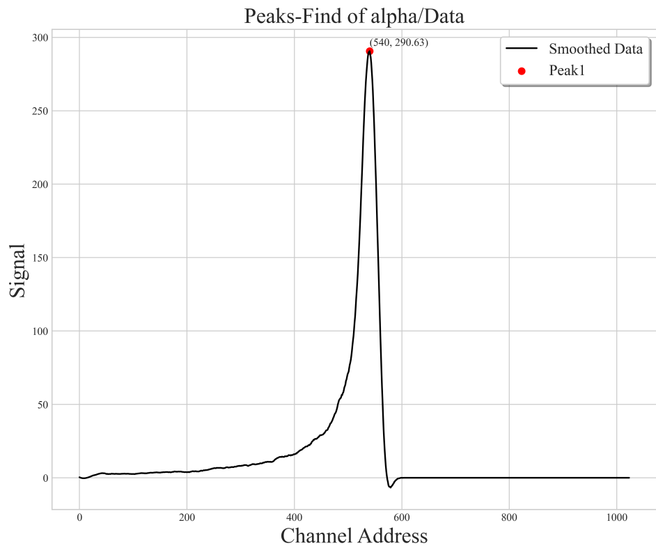
图 11: ^{241}\text{Am} 能谱通过 Al 膜后的滤波处理 + 寻峰
