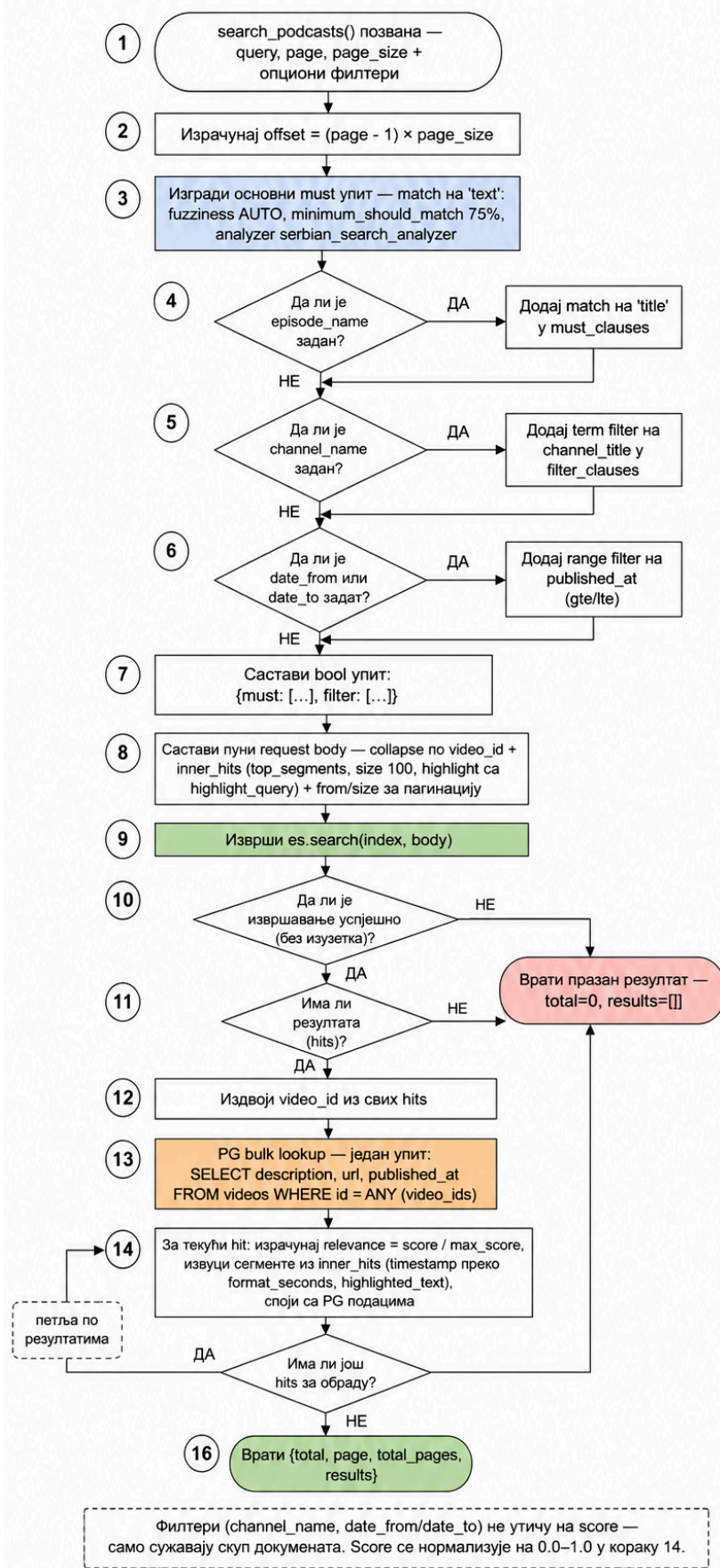
Слика 7: Алгоритам корисничке претраге у Elasticsearch-у
