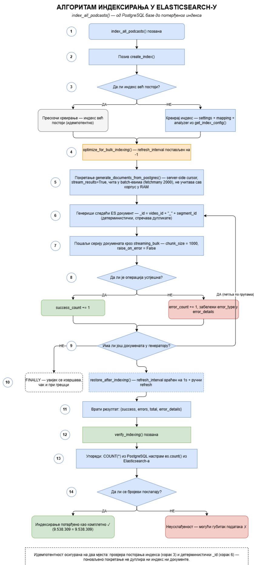
Слика 6: Алгоритам индексирања у Elasticsearch-у
