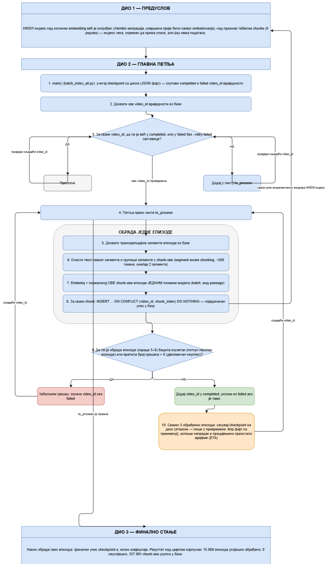
Слика 8: Алгоритам batch embed -овања корпуса и уписа векторских репрезентација у базу
