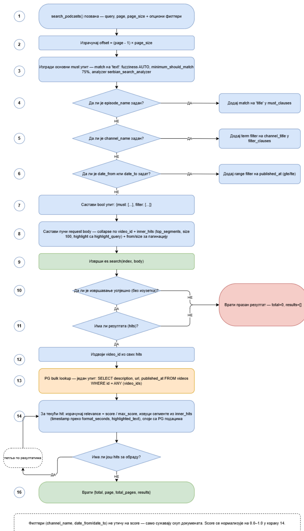
Слика 7: Алгоритам корисничке претраге у Elasticsearch-у
