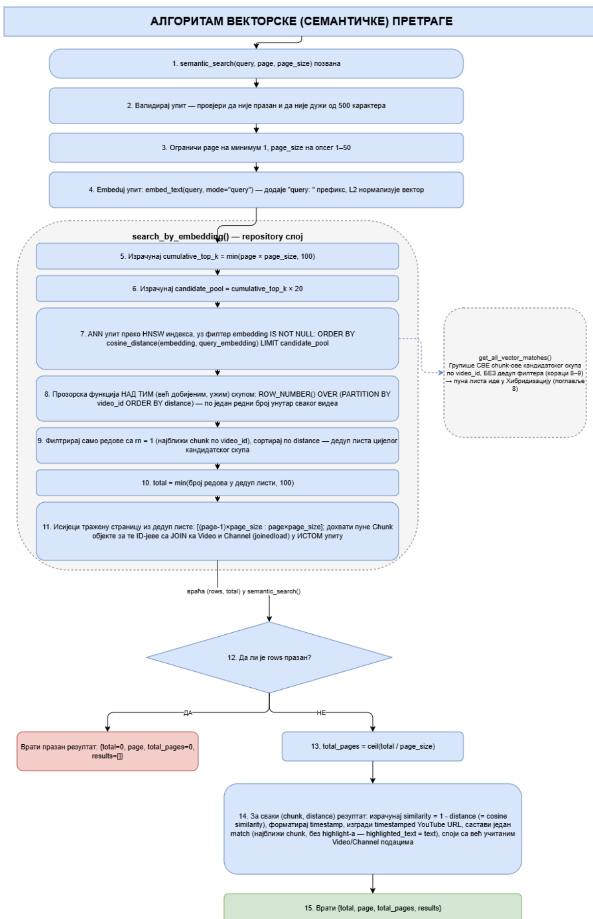
Слика 9: Алгоритам векторске претраге
