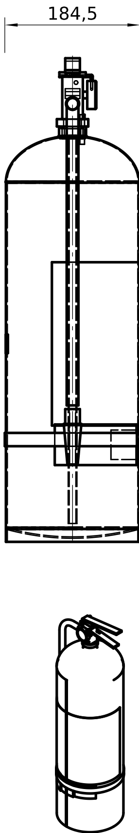
ISOMETRÍA (ESC. 1:10)
