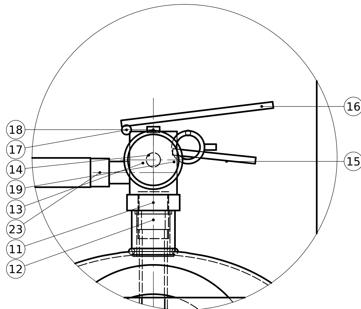
DETALLE A (1:2) Válvula, manómetro y manijas
