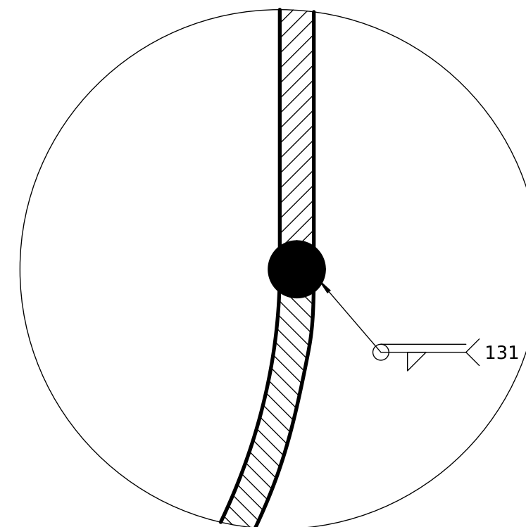
DETALLE D (2:1) Unión fondo-cuerpo
