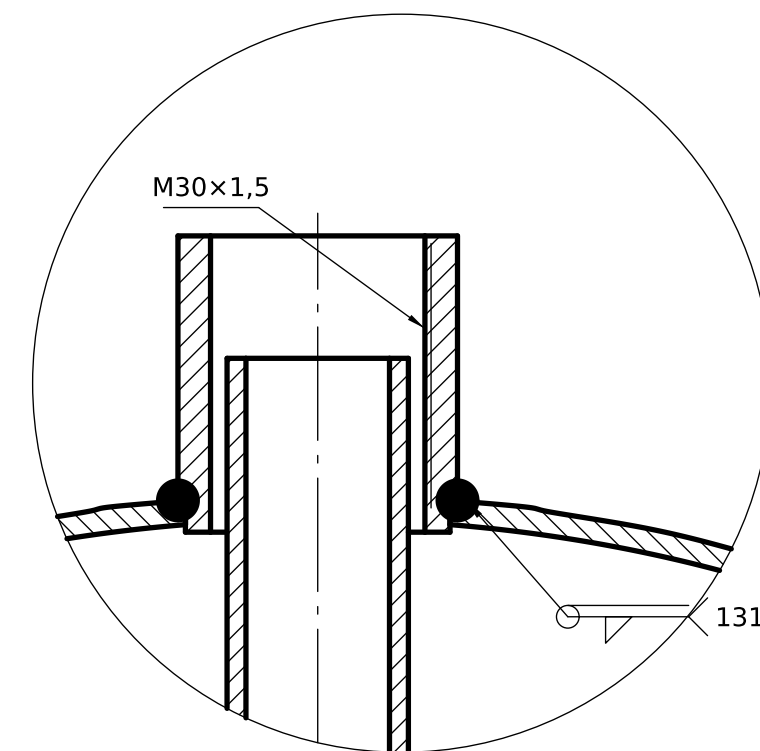
DETALLE B (1:1) Cuello roscado
