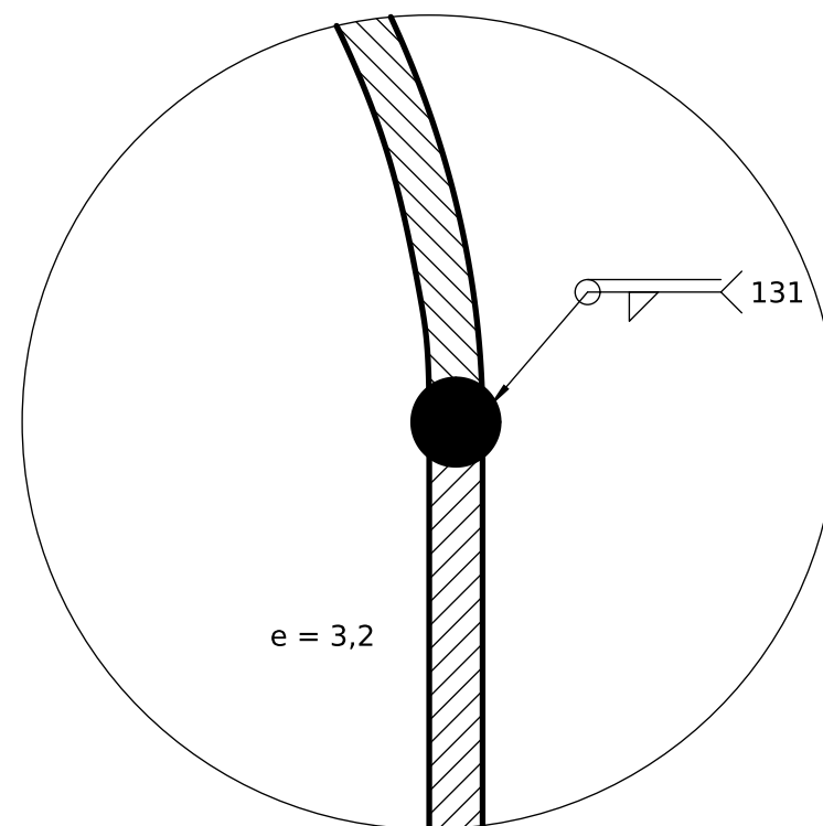
DETALLE C (2:1) Unión cúpula-cuerpo
