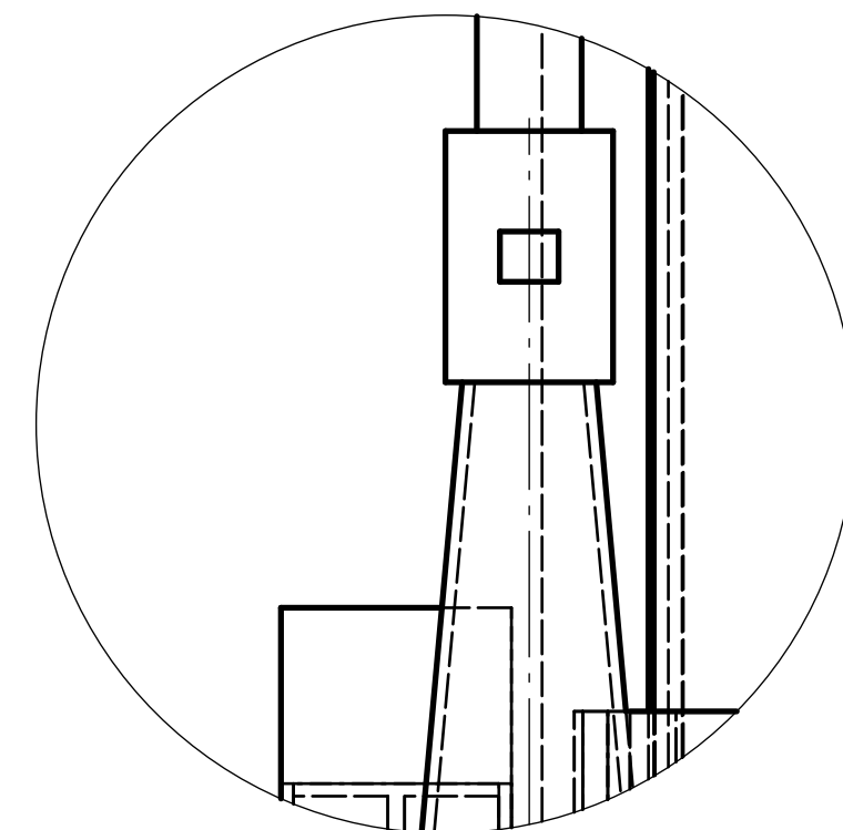
DETALLE E (1:2) Válvula esférica y tobera
