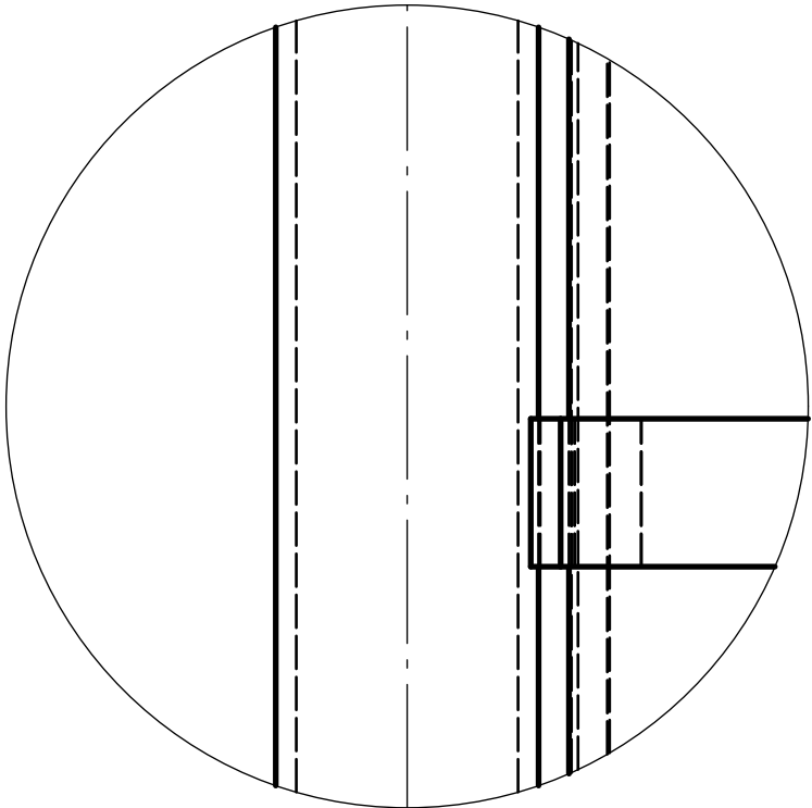
DETALLE E (1:1) Lanza espumígena
