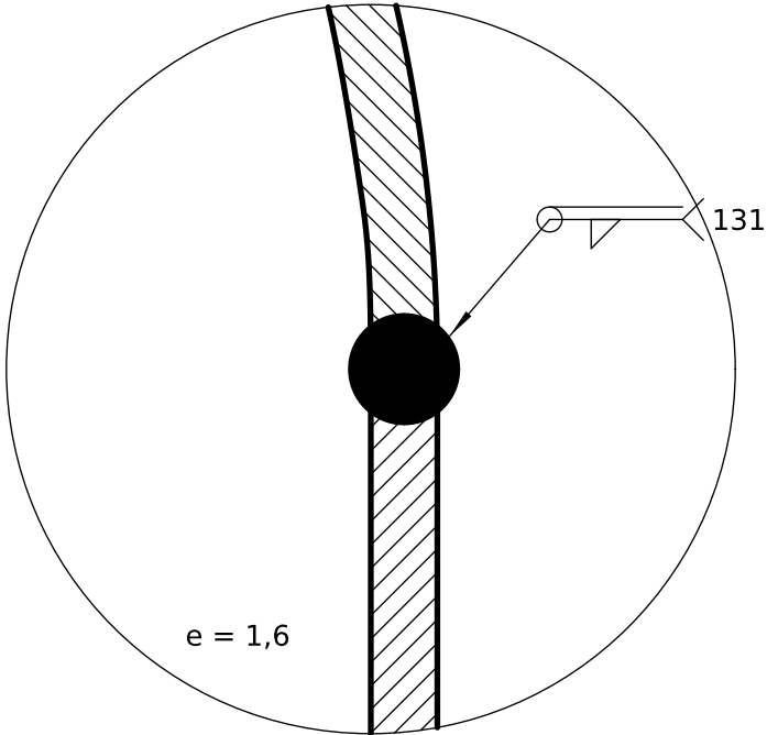
DETALLE C (5:1) Unión cúpula-cuerpo
