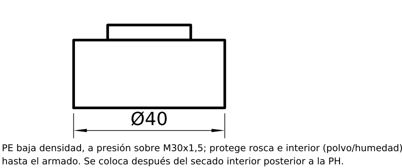
R4 TAPÓN PROTECTOR DE ROSCA
