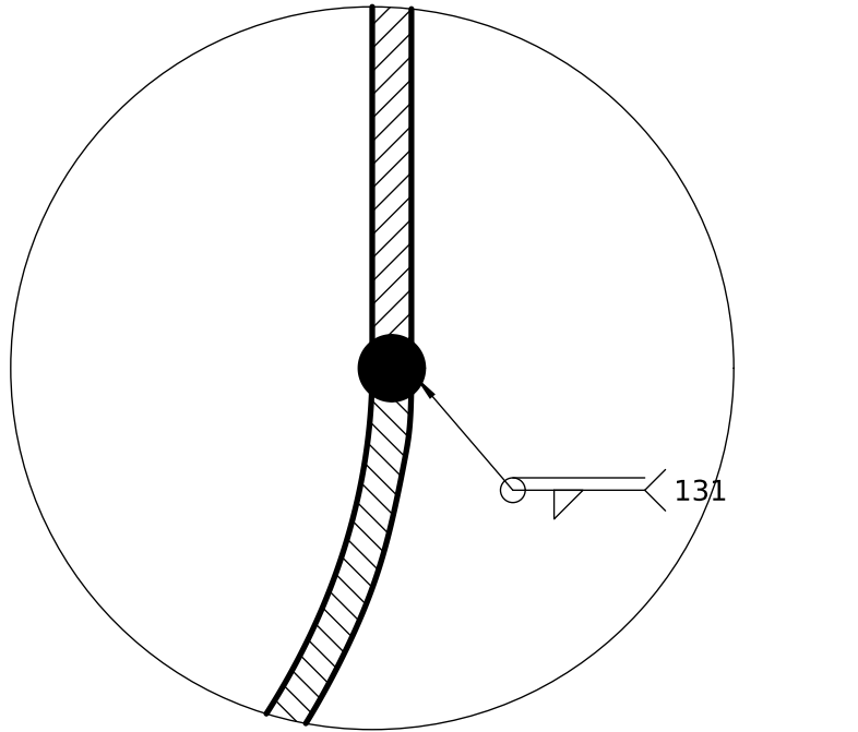
DETALLE D (1:1) Unión fondo-cuerpo
