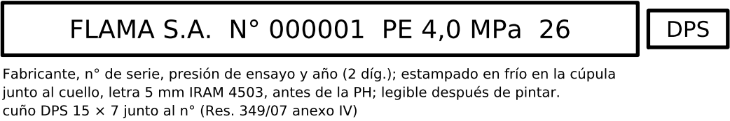
R3 MARCADO GRABADO (IRAM 3550 5.1)
