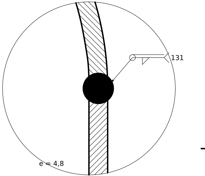
DETALLE C (2:1) Unión cúpula-cuerpo
