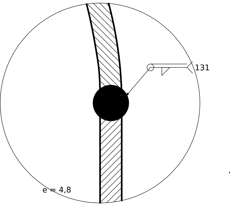
DETALLE C (2:1) Unión cúpula-cuerpo
