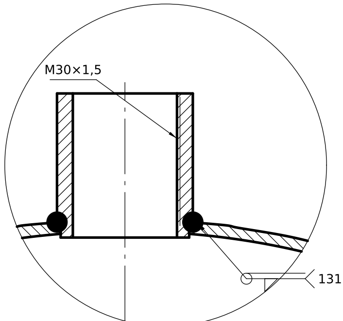
DETALLE B (1:1) Cuello roscado
