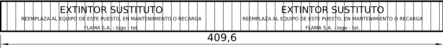
DETALLE 1 - DESARROLLO DE LA FAJA 28 × 410 (esc. 1:2) - amarillo; leyendas negras repetidas
