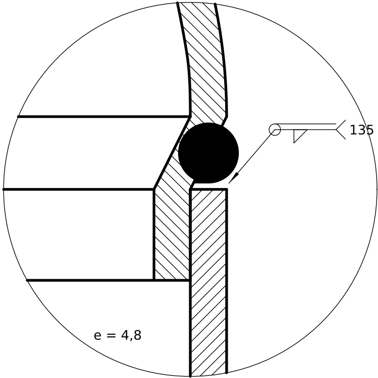
DETALLE C (2:1) Casquete con borde reducido y tope
