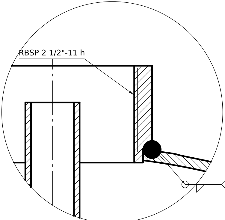
DETALLE B (1:1) Cupla soldada
