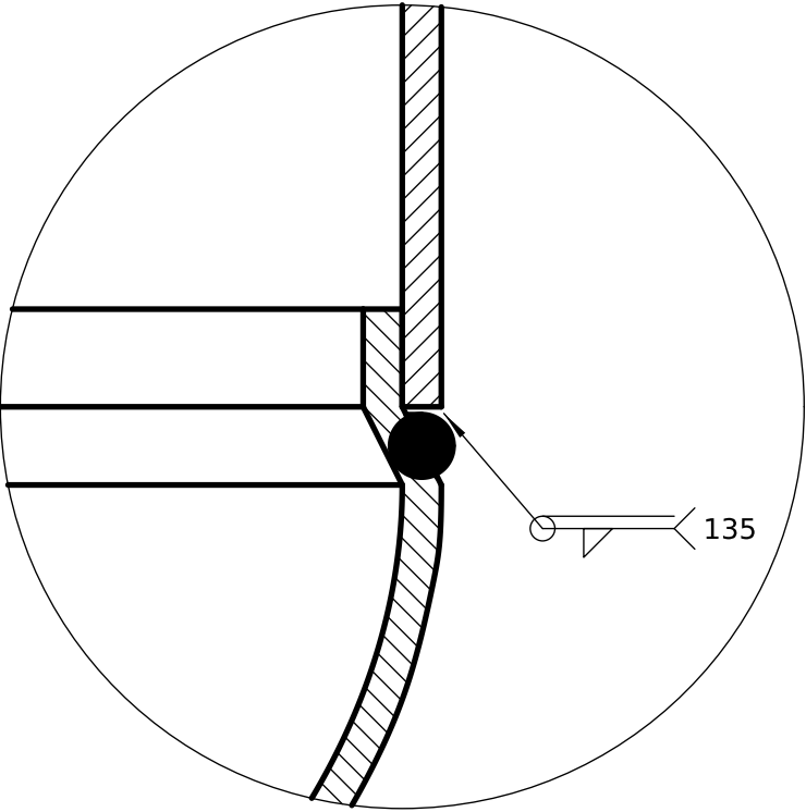
DETALLE D (1:1) Casquete inferior con borde reducido
