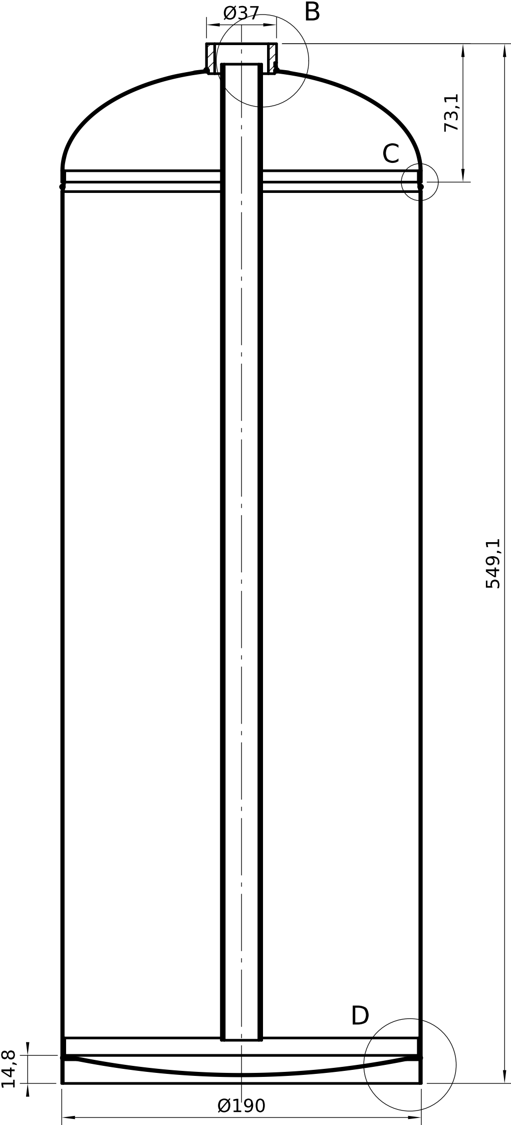
CORTE A-A (1:2)
