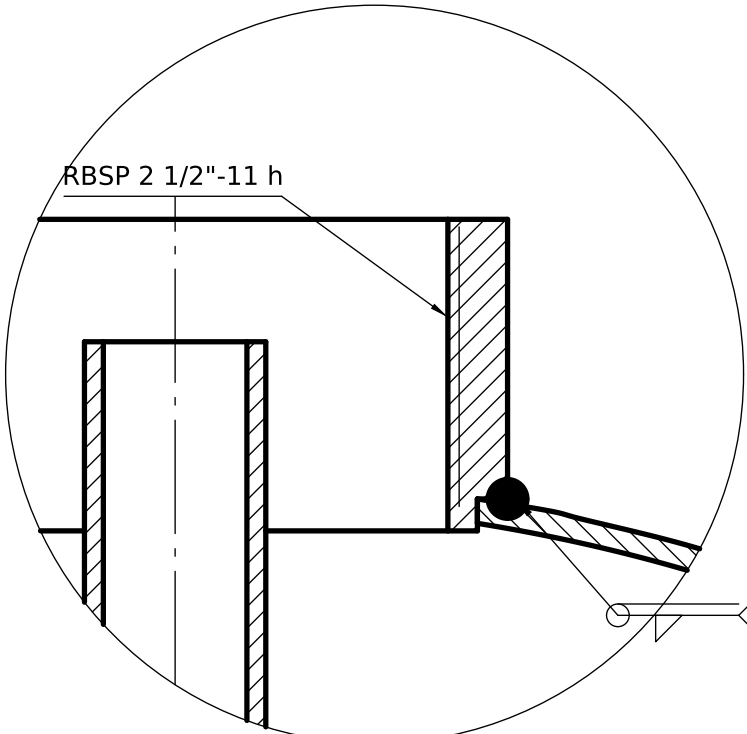
DETALLE B (1:1) Cupla soldada
