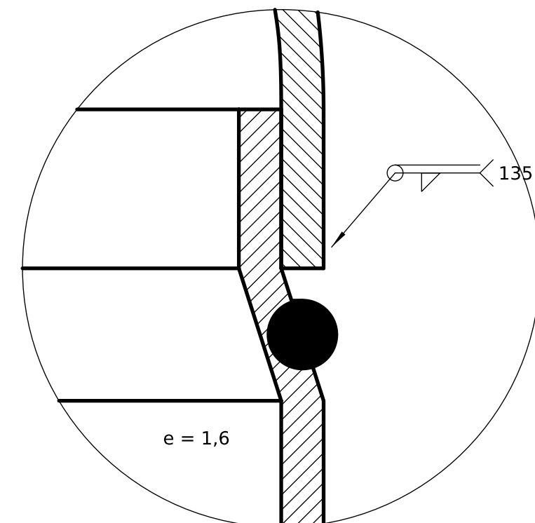
DETALLE C (5:1) Bordón del cuerpo y cúpula
