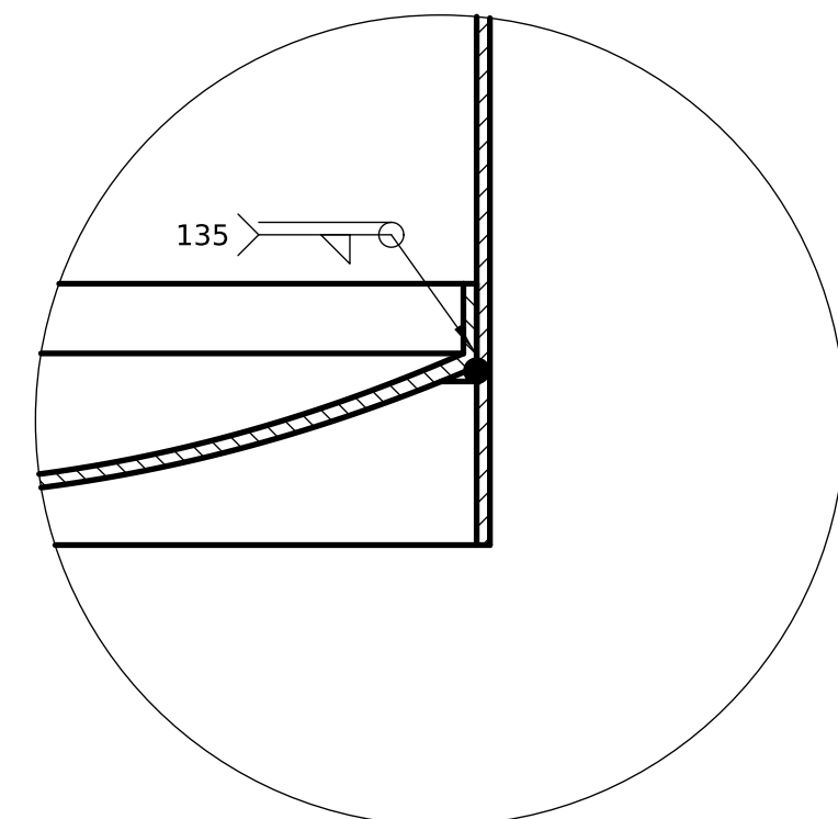
DETALLE D (1:1) Fondo encastrado y pollera
