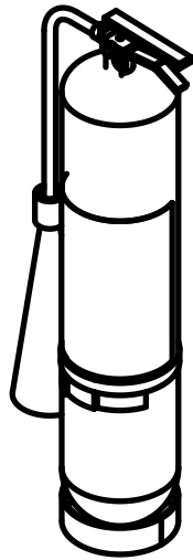
ISOMETRÍA (ESC. 1:10)
