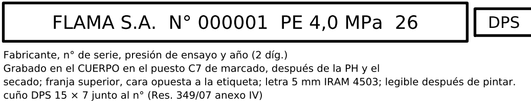
R3 MARCADO GRABADO (IRAM 3550 5.1)
