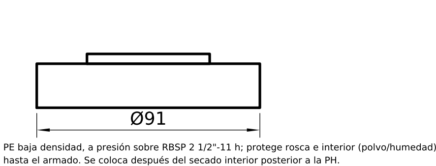
R4 TAPÓN PROTECTOR DE ROSCA
