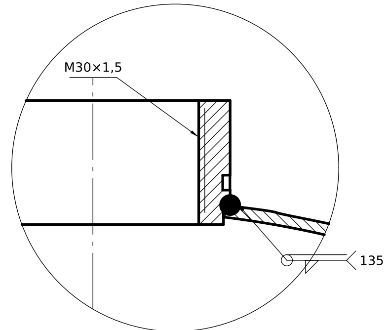
DETALLE B (2:1) Cuello roscado muesca de altura 2 x 1 x 2 (prensa Pannier); filete exterior
