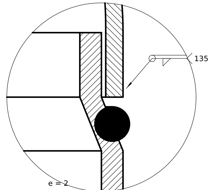
DETALLE C (5:1) Bordón del cuerpo y cúpula escalón e 2 x 5, labio 6 (bordoneadora); cúpula por fuera
