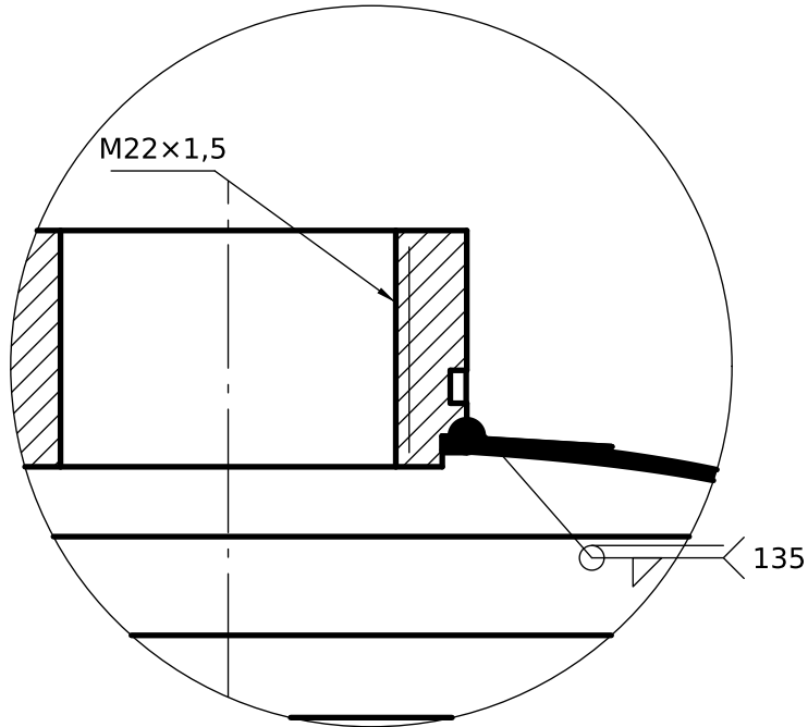
DETALLE B (2:1) Cuello roscado muesca de altura 2 x 1 x 2 (prensa Pannier); filete exterior
