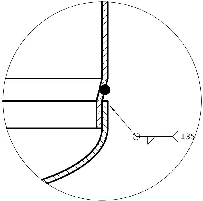
DETALLE D (2:1) Bordón inferior y fondo caño con los dos extremos reducidos: escalón e 1,25 x 5, labio 6
