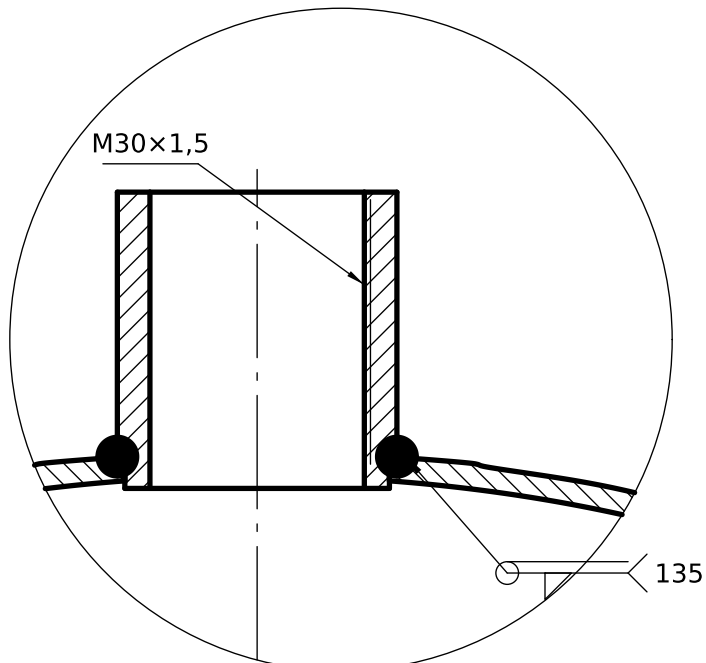
DETALLE B (1:1) Cuello roscado cupla soldada por fuera con filete (posicionador)
