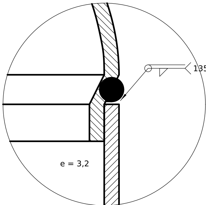
DETALLE C (2:1) Casquete con borde reducido y tope labio 8 dentro del cuerpo, escalón 6,4 x e 3,2; cordón en el escalón
