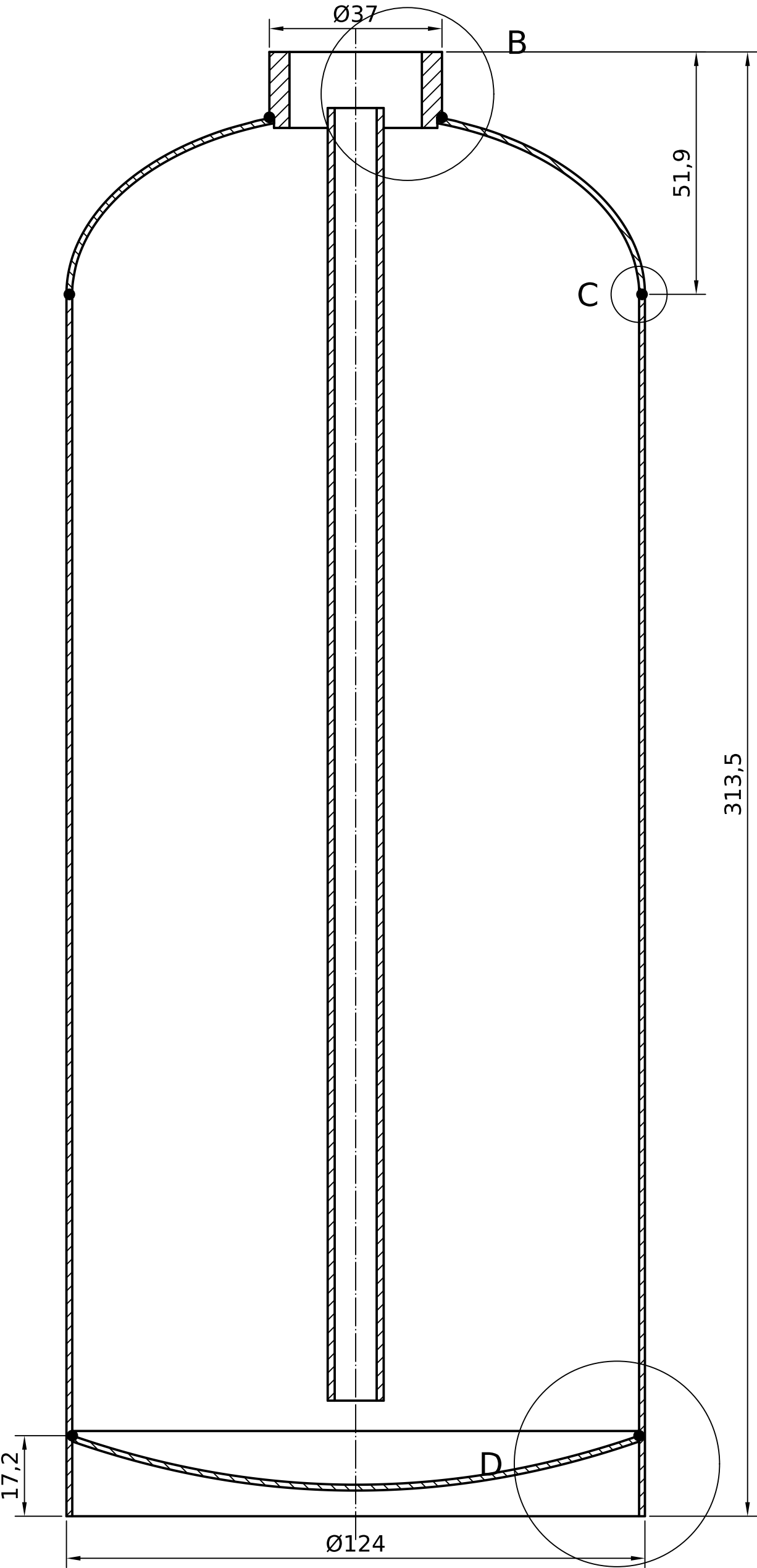
A-A (1:1)
