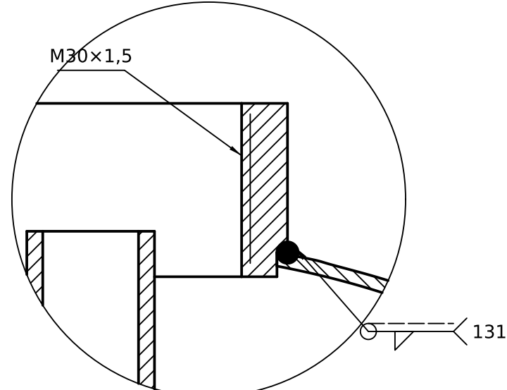
B (2:1) Cuello roscado
