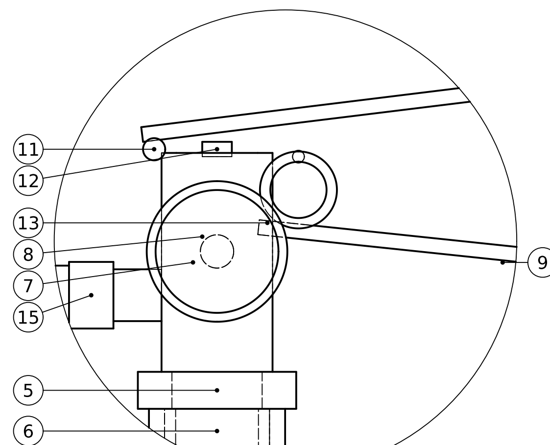
A (1:1) Válvula, manómetro y manijas
