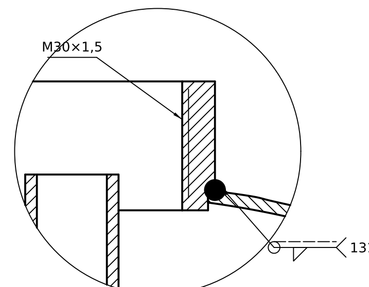
B (2:1) Cuello roscado
