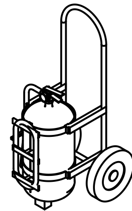
ISOMETRÍA (1:20)
