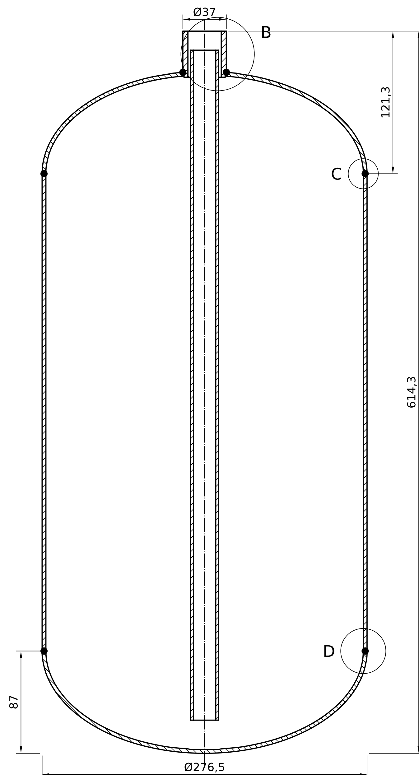
A-A (1:2)
