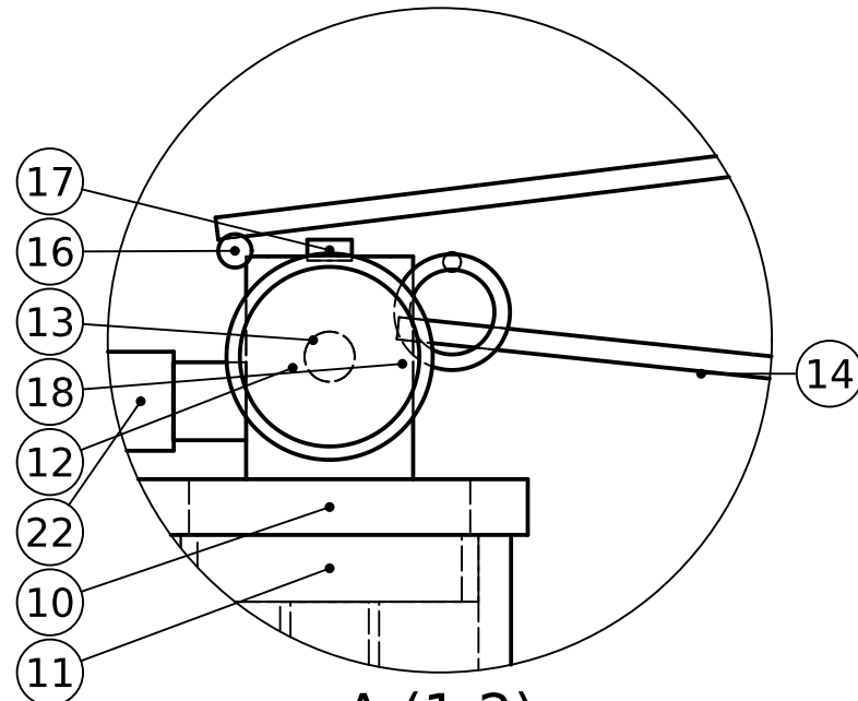
A (1:2) Válvula, manómetro y manijas
