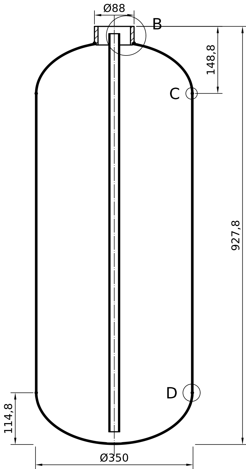
A-A (1:5)
