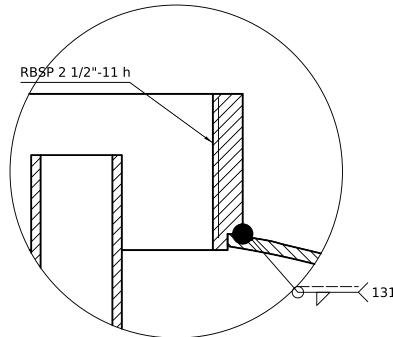
B (1:1) Cuello roscado
