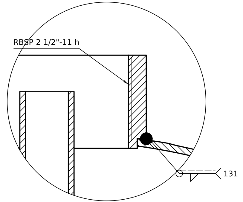
B (1:1) Cuello roscado
