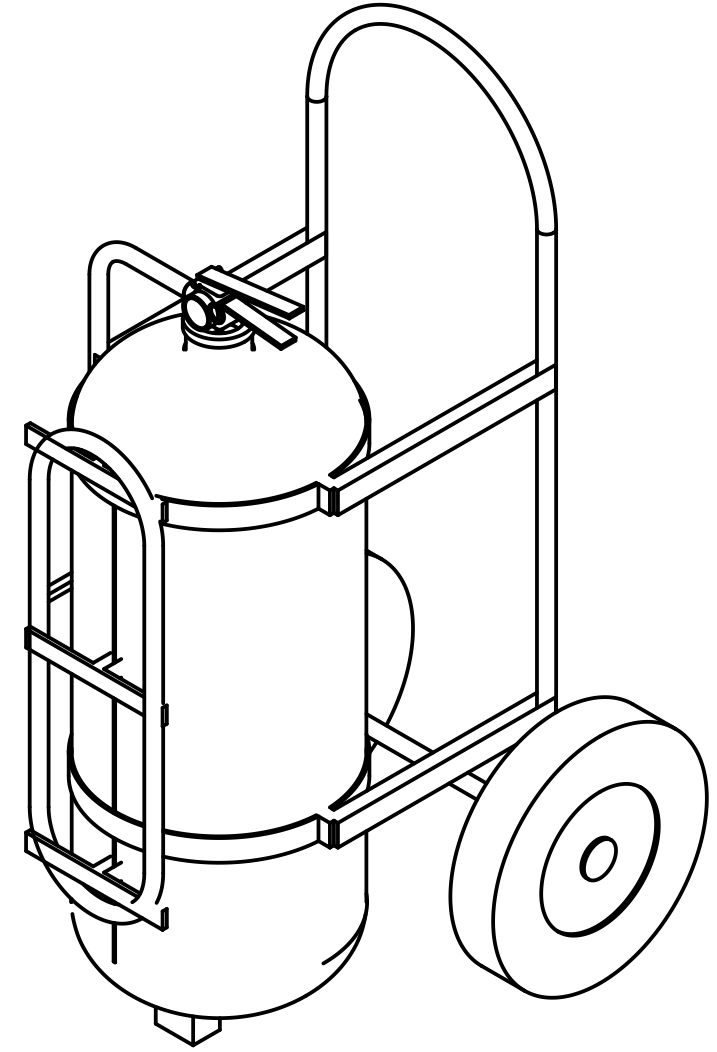
ISOMETRÍA
