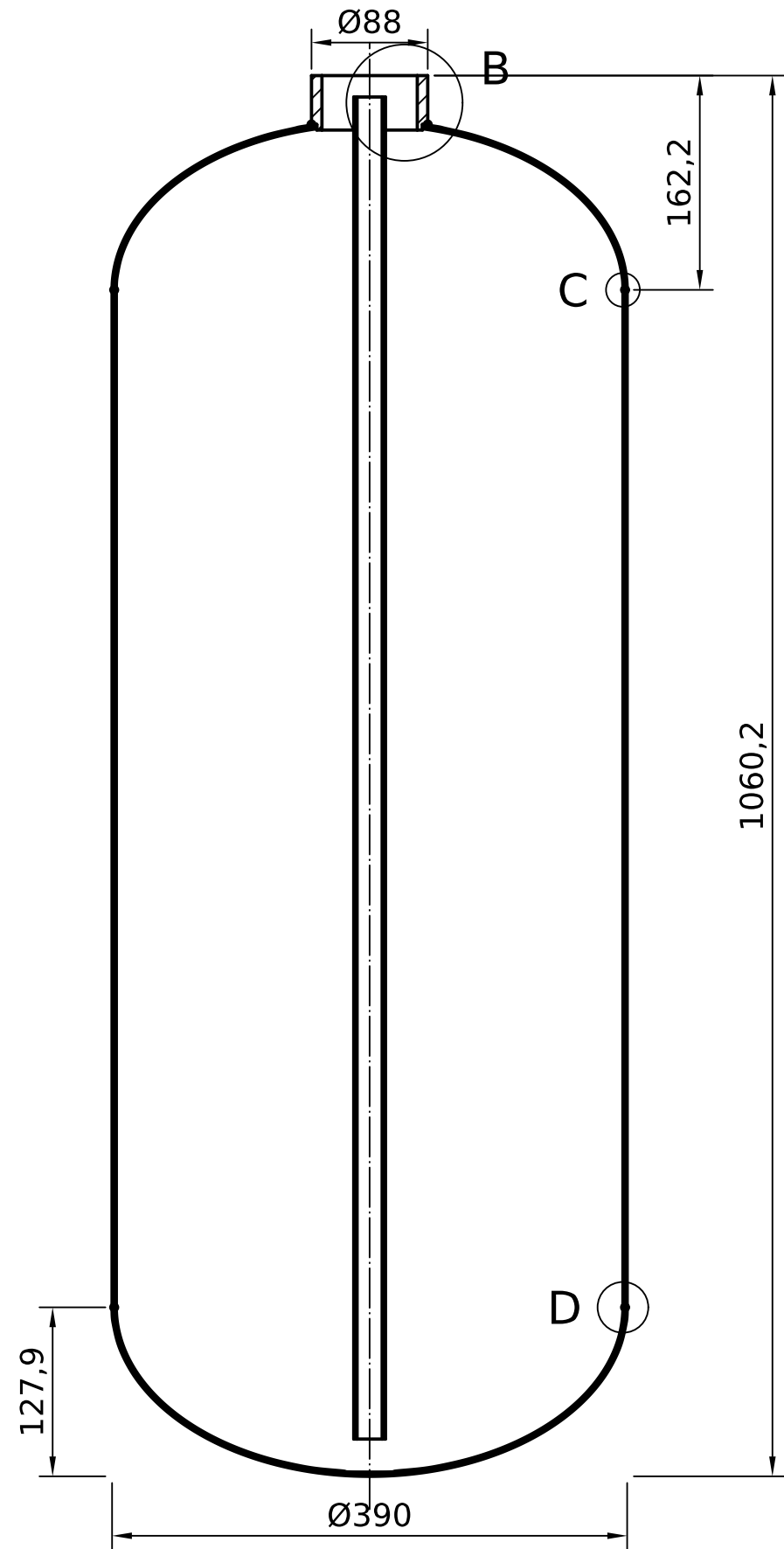
A-A (1:5)
