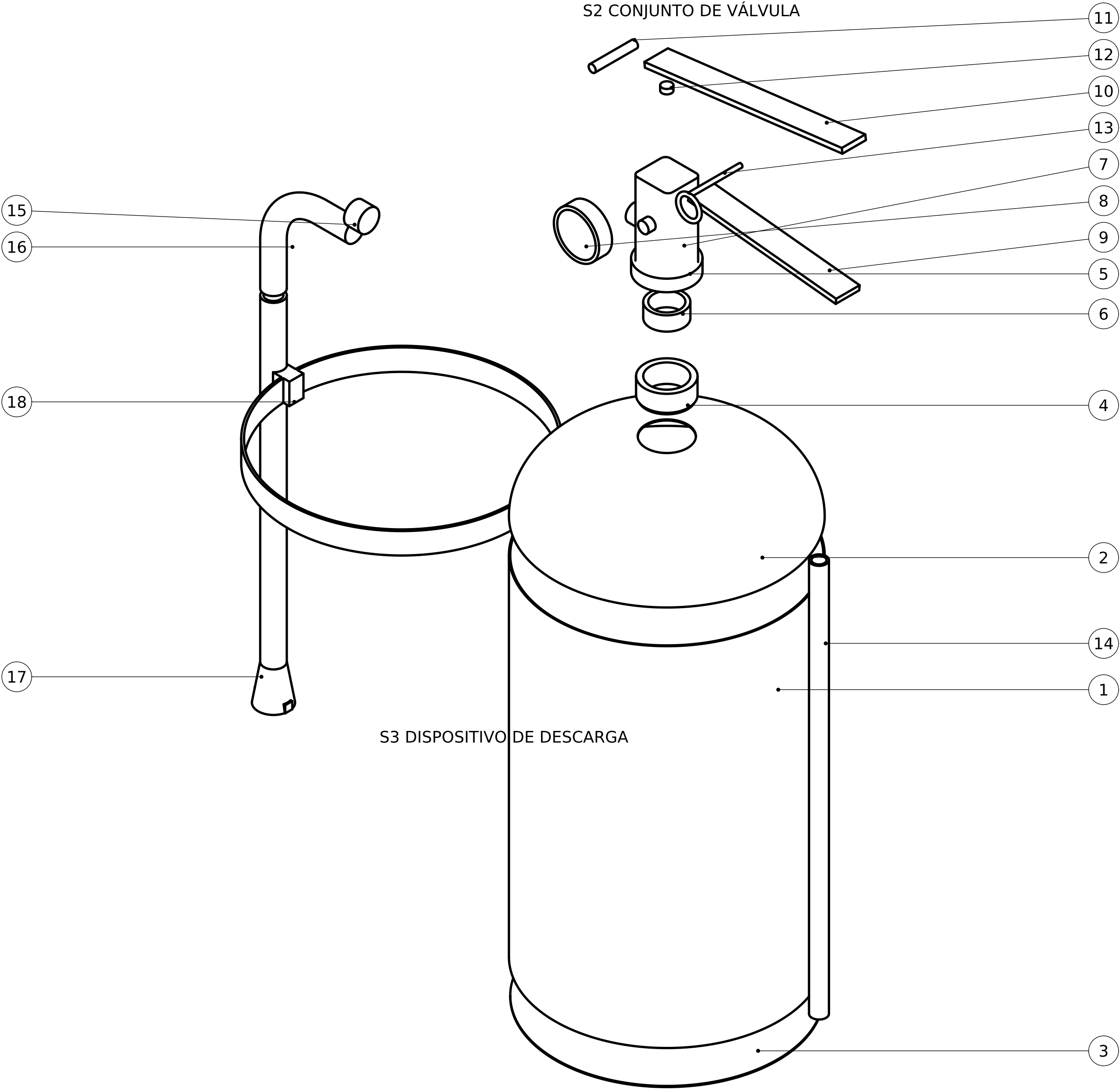
S2 CONJUNTO DE VÁLVULA
