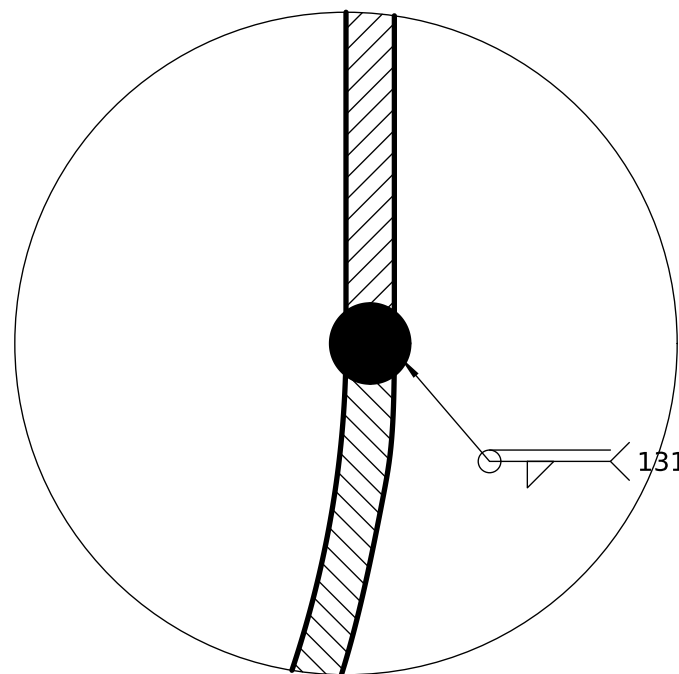
DETALLE D (2:1) Unión fondo-cuerpo
