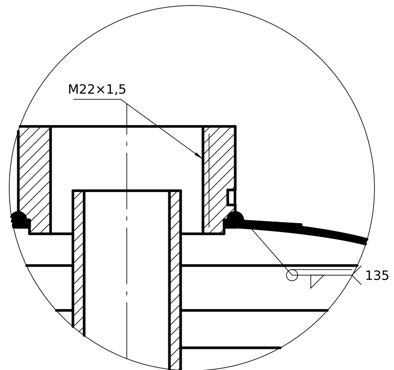
DETALLE B (2:1) Cuello roscado con muesca
