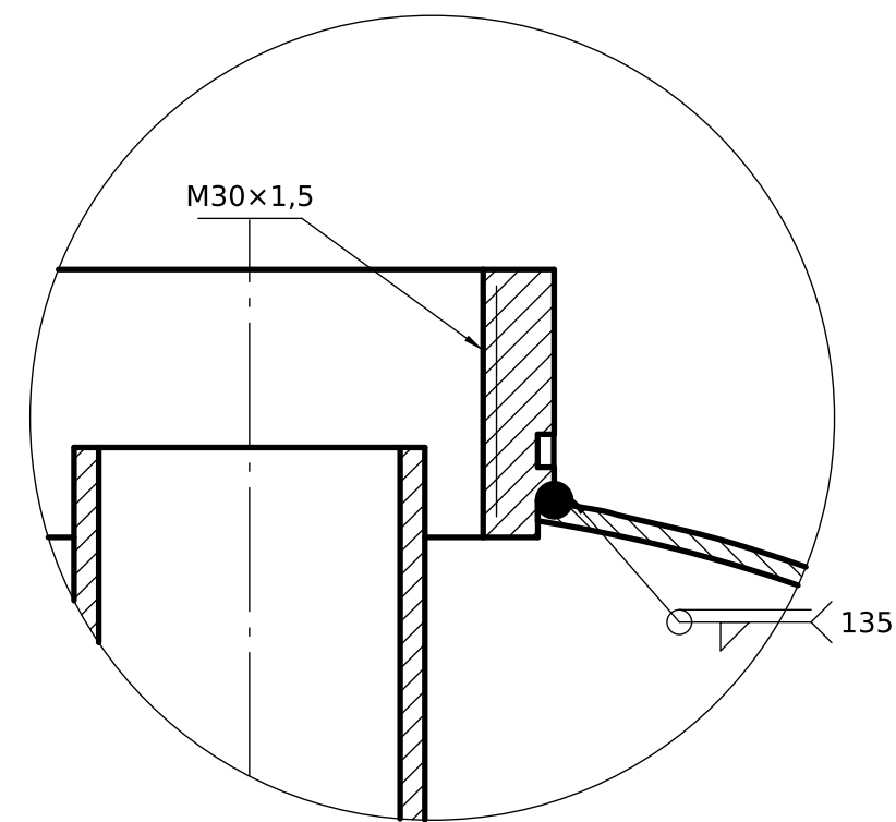
DETALLE B (2:1) Cuello roscado con muesca
